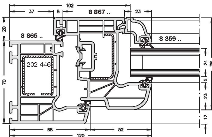
Combinación de perfiles estándar; E. 1:2
