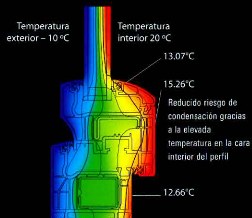
Corona CT 70 Termografía de la sección
